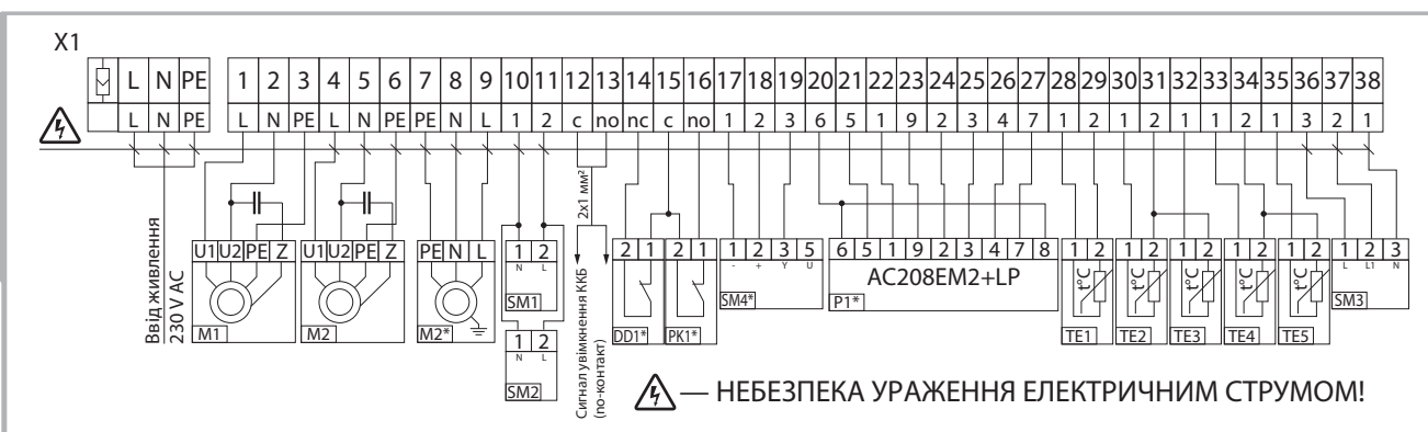
Мал. 18. Схема зовнішніх підключень ВУТ 1500 (2000) ВГ
