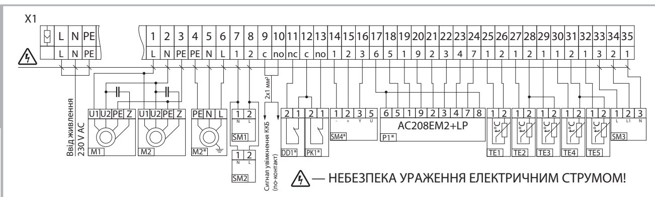
Мал. 17. Схема зовнішніх підключень ВУТ 800 (1000) ВГ
