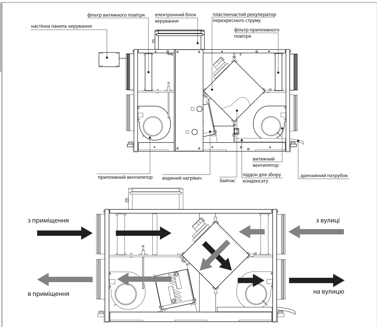
Мал. 10. Будова та принцип роботи установки
