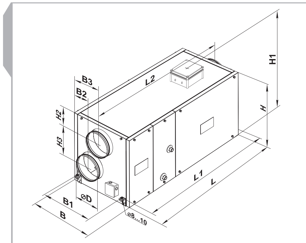
Мал. 1. Габаритні та приєднувальні розміри
